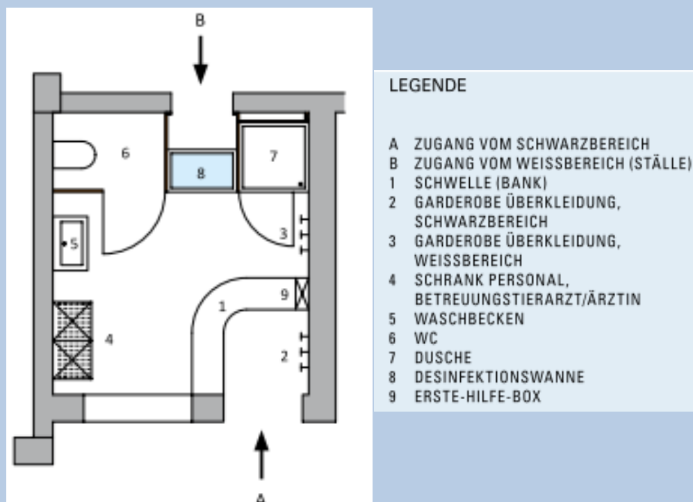
Abbildung 4: Hygieneschleuse ; Landwirtschaftskammer OÖ Abteilung Bildung und Beratung.
