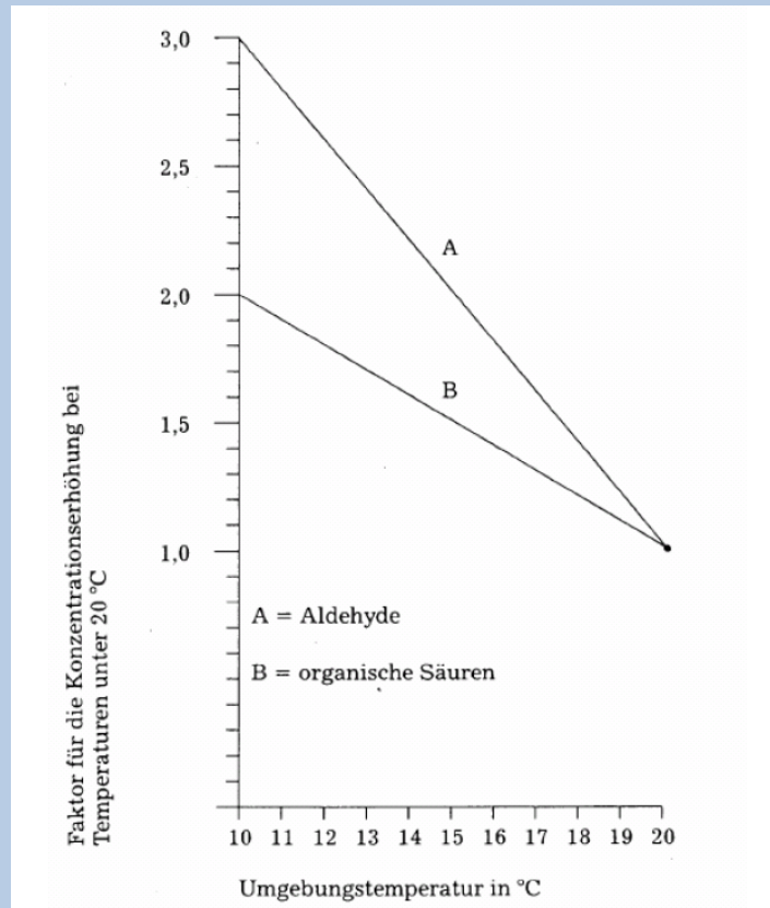
Abbildung 3: Temperaturabhängige Konzentrationserhöhung aus: Richtlinie des Bundesministeriums für Ernährung, Landwirtschaft und Verbraucherschutz über Mittel und Verfahren für die Durchführung der Desinfektion bei anzeigepflichtigen Tierseuchen (323-35130/0001, Stand Februar 2007)
